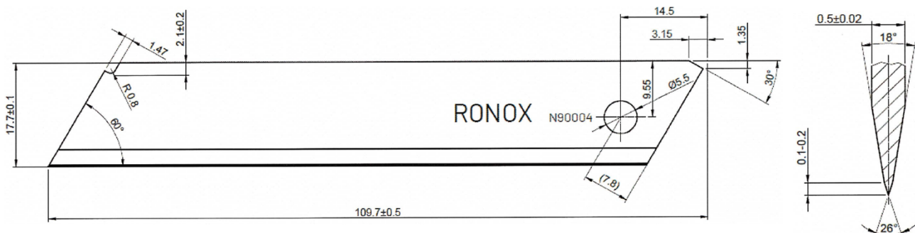
Geometria szlifu
