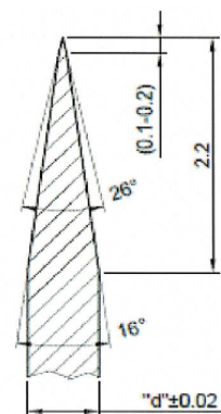
Geometria szlifu
