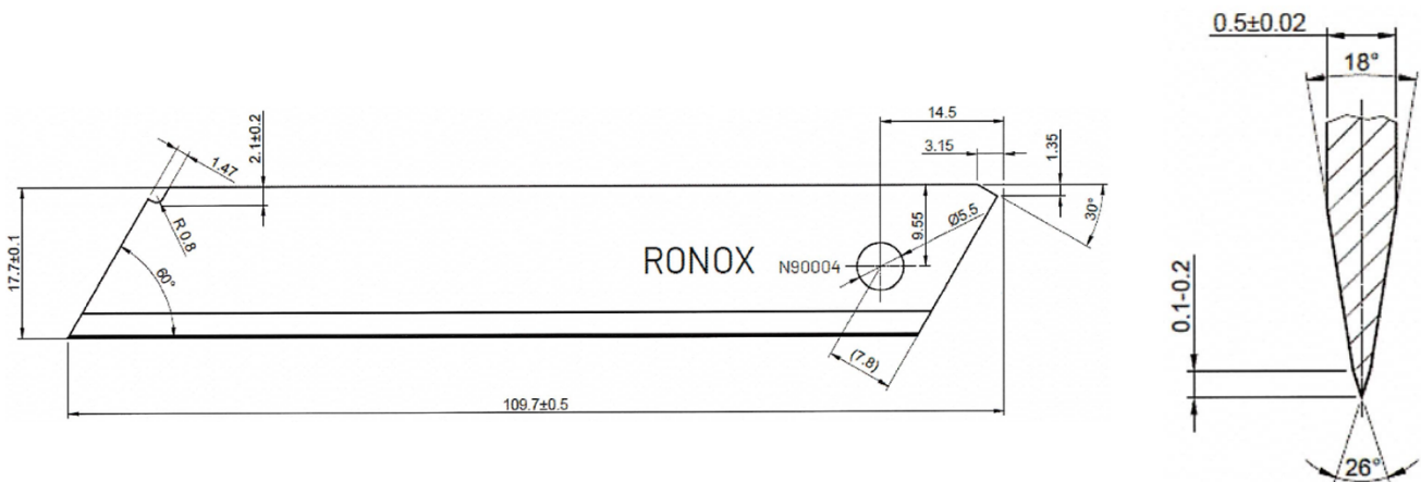
Geometria szlifu
