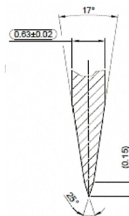
Geometria szlifu
